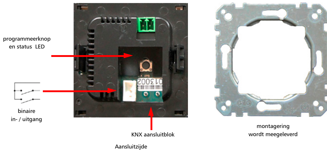
SK30-XX-inbouw informatie
