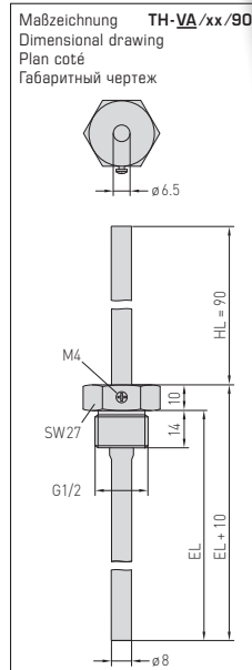
TF 54 + TH-xx/90 Edelstahltauchhülse mit Halsrohr Stainless steel immersion sleeve with neck tube doigt de gant en acier inox avec tube prolongateur Гильза погружная из высококачественной стали с горловиной
