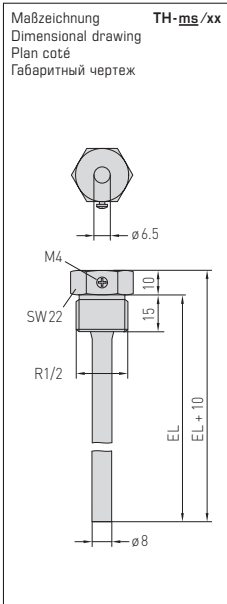
TF 54 + TH-ms/xx Messingtauchhülse Brass immersion sleeve doigt de gant en laiton Гильза погружная из латуни
