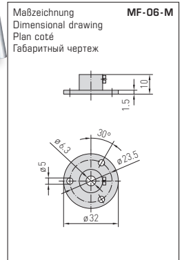
MF-06-M Montageflansch aus Metall Mounting flange, metal Bride de montage en métal Присоединительный фланец из металла
