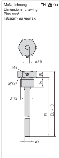
TF 54 + TH-VA/xx Edelstahltauchhülse Stainless steel immersion sleeve doigt de gant en acier inox Гильза погружная из высококачественной стали
