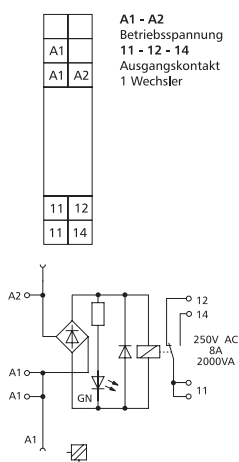
Aansluitschema / schakelschema
