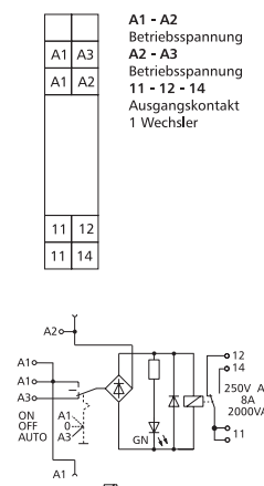
Aansluitschema / schakelschema
