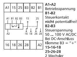
Aansluitschema / schakelschema
