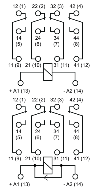
Aansluitschema
