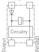
Одиночное подключение
