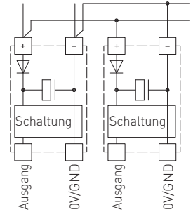
Parallelbetrieb
