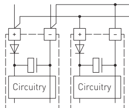
Параллельное подключение
