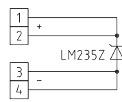
1x vierdraadsschakeling LM235 Z (KP 10)
